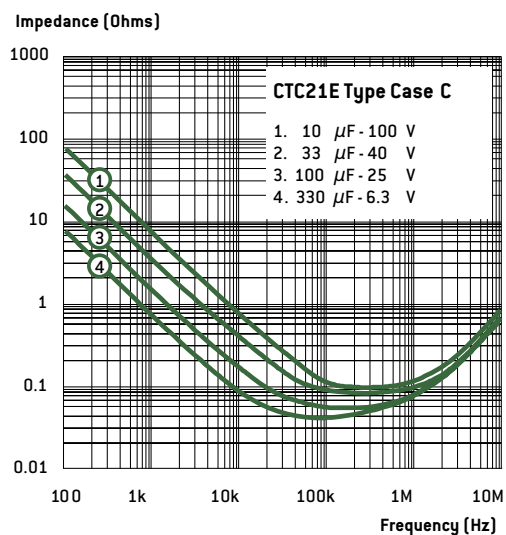
CTC21E TYPE CASE C
